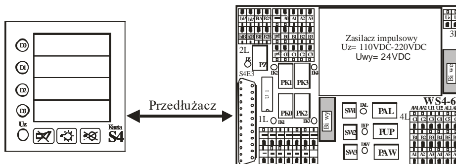
Rys. 15 Schemat połączeń zewnętrznych kasyety S4-E3P z listwą WS4-6
