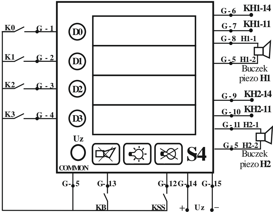
Rys. 2 Schemat połączeń zewnętrznych kasy S4-E3, zasilanie wejść napięciem COM
