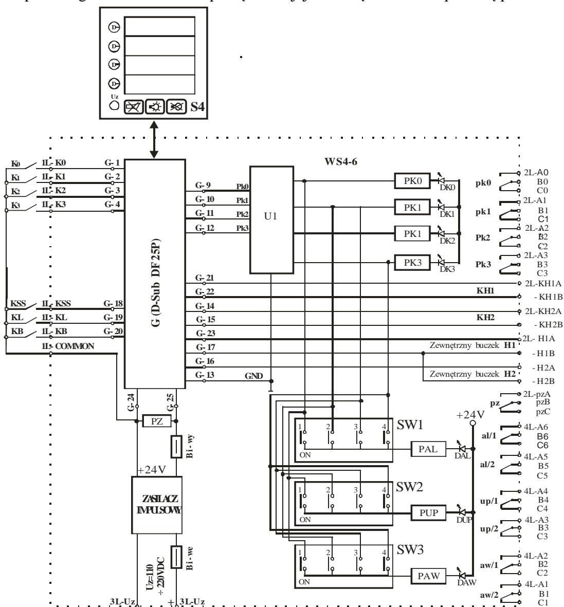
Rys. 16 Schemat blokowy listwy pośredniej WS4-6 i schemat połączeń zewnętrznych
