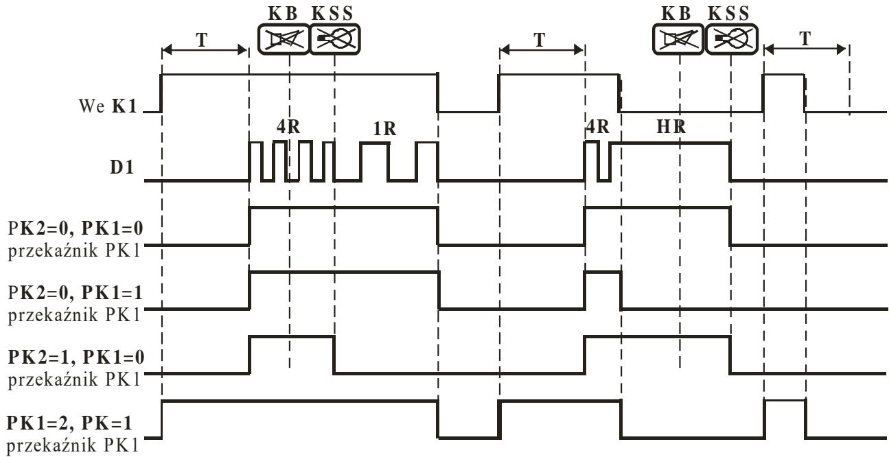
Rys. 10 Przebieg czasowy reakcji listwy WS4-6
