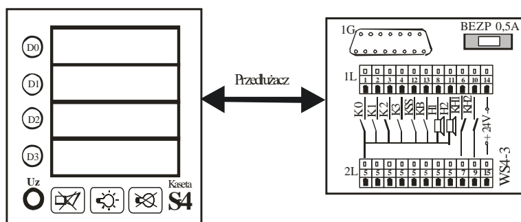
Rys. 13 Schemat połączeń zewnętrznych kasyety S4-E3 z listwą WS4-3
