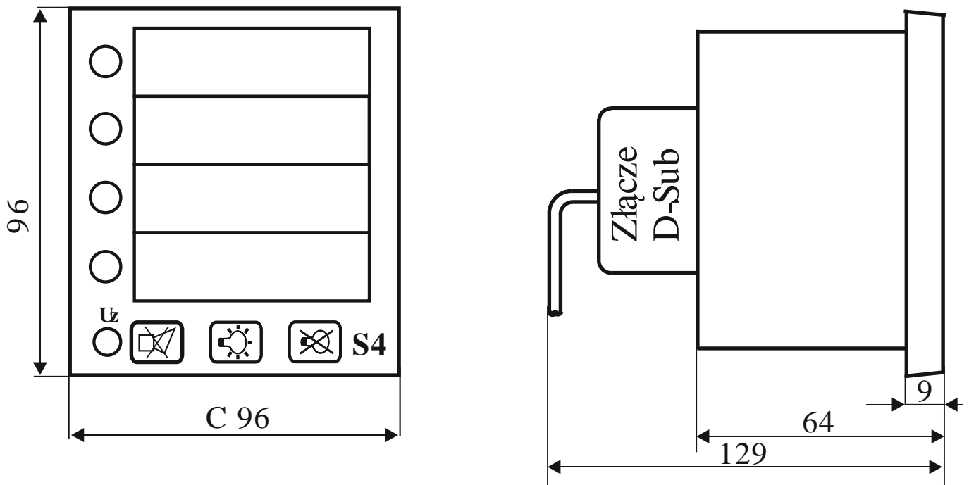
Rys. 1 Wymiary kasety S4-E3
