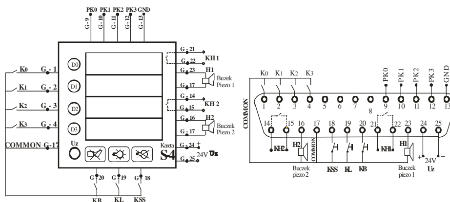
Rys. 14 Schemat połączeń zewnętrznych i opis gniazda przyłączeniowego G kasyety S4-E3P
