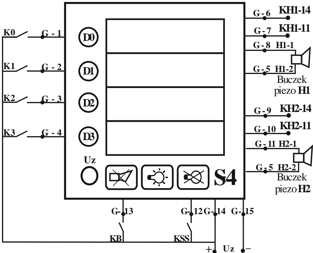
Rys. 3 Schemat połączeń zewnętrznych kasy S4-E3, zasilanie wejść napięciem + Uz
