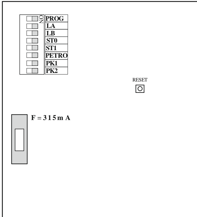
Rys. 5 Programowanie kasety S4-E3 wewnątrz kasety
