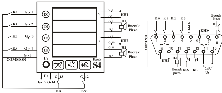
Rys. 11 Schemat połączeń zewnętrznych i opis gniazda przyłączeniowego G kasety S4-E3 z wykorzystaniem napięcia COMMON
