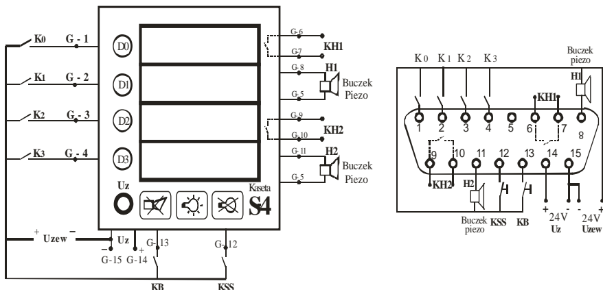
Rys. 11 Schemat połączeń zewnętrznych i opis gniazda przyłączeniowego G kasety S4-E3 z wykorzystaniem napięcia COMMON
