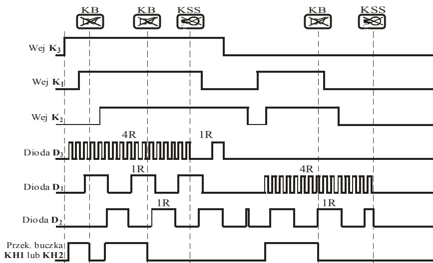
Rys.7 Przebieg czasowy funkcji wyróżnienia pierwszego sygnału
