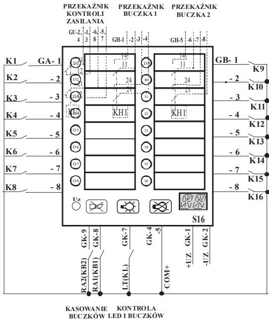
Rys.9 Schemat połączeń zewnętrznych i opis gniazd przyłączeniowych kasyety-S16B(A)-E4w
