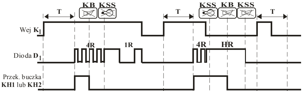
Rys.3 Przebieg czasowy funkcji awaryjnej z pamięcią, z czasem opóźnienia T
