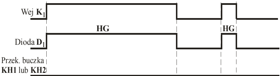
Rys.4 Przebieg czasowy funkcji powtarzacza
