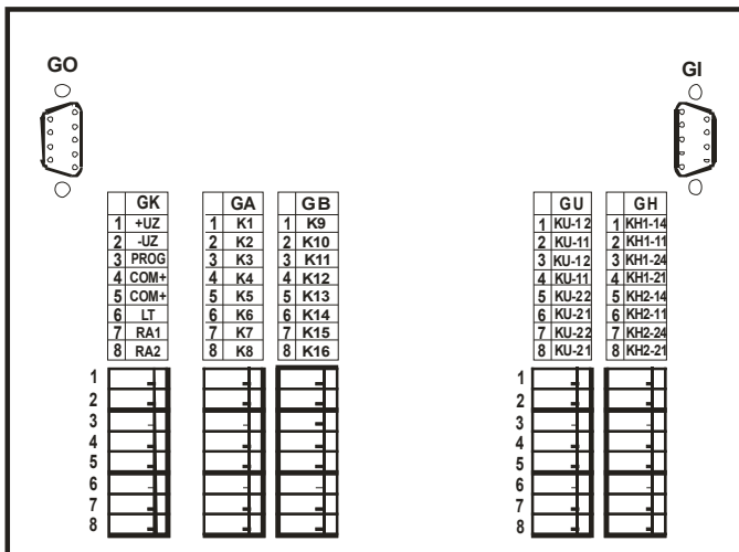
Rys.11 Opis gniazd przyłączeniowych kasety S16B-E4w
