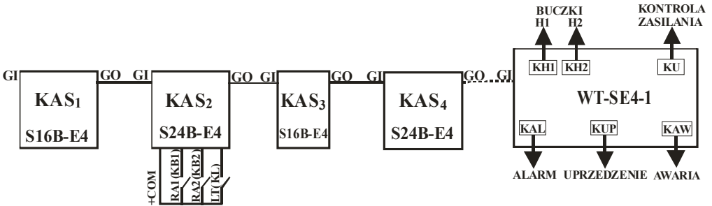
Rys.12 Łączenie kaset E4 w grupy
