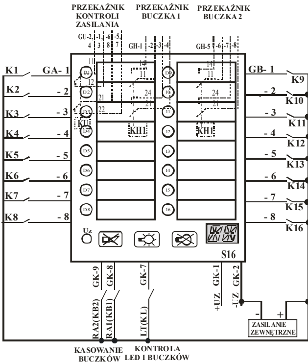
Rys.10 Schemat połączeń zewnętrznych i opis gniazd przyłączeniowych kasety-S16B(A)-E4w z wykorzystaniem napięcia zewnętrznego Uzew
