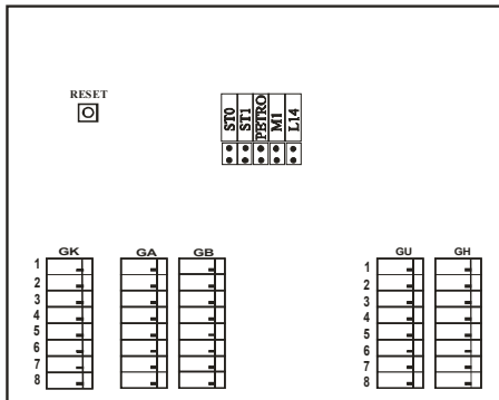
Rys.2 Obszar programowania całej kasety
