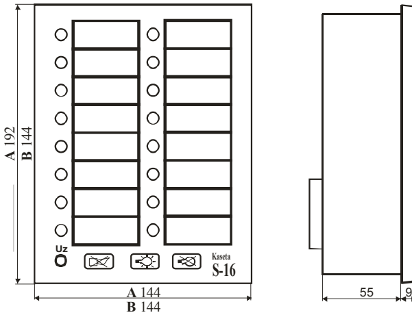
Rys.8 Wymiary kasyety S16B(A)-E4
