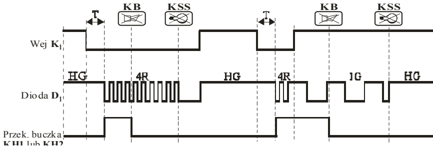
Rys.5 Przebieg czasowy funkcji kontroli pracy silnika lub pompy PETRO=0
